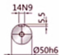
入力軸
